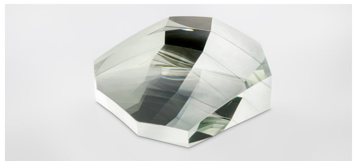
Prisma für das Projekt EnMAP*.
